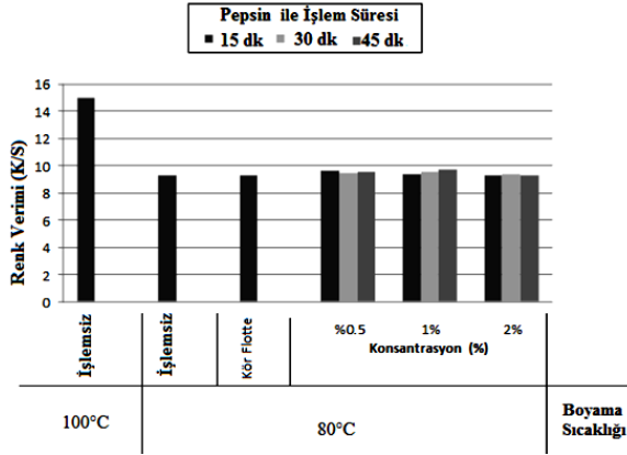
Şekil 5: Aspartik tipi proteaz ile çeşitli koşullarda ön işlemin ipek liflerinin boyanmasında elde edilen renk verimi üzerine etkisi
