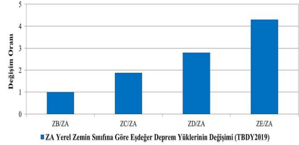
Şekil 5. ZA zemin sınıfına göre eşdeğer deprem yüklerinin değişimi
